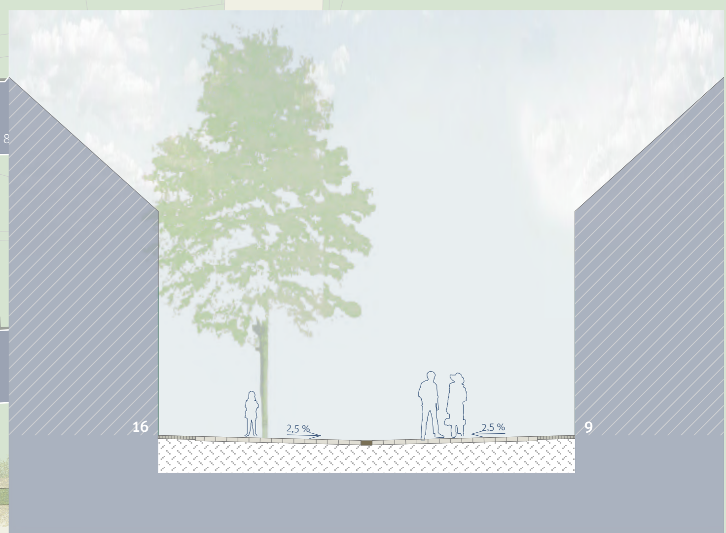
Schnitt B - B | M 1:100
